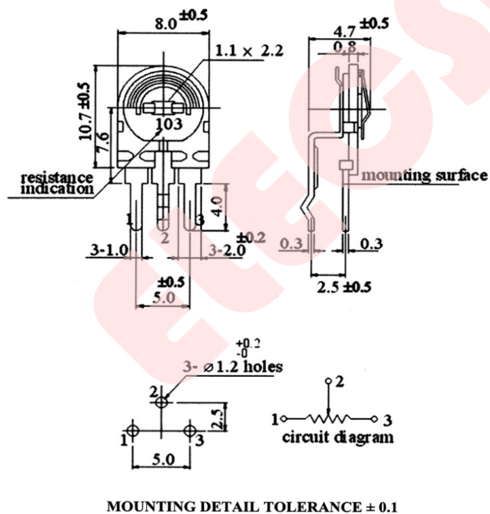
STYLE : ET085-E
