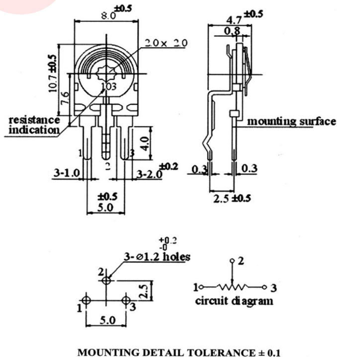
STYLE : ET085-F
